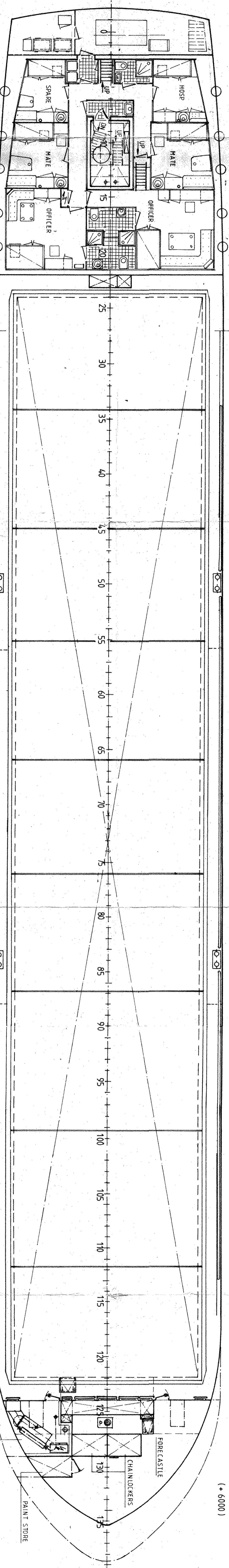
MAINDECK / HOOFDDECK (1-6000)
